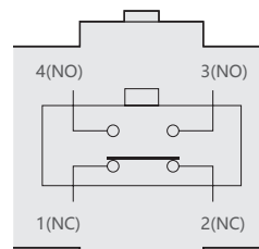
Расположение контактов
